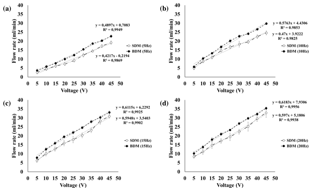
Fig. 9. Maximum flow rate results at (a) 5 Hz, (b) 10 Hz, (c) 15 Hz and (d) 20 Hz.
